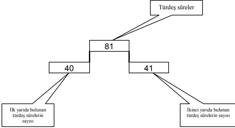
Şekil-16 Türdeş sûrelerin (asal-asal değil) dağılımı görülmüyor.
