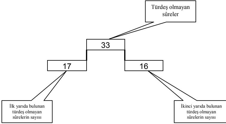
Şekil-17 Türdeş olmayan sûrelerin (asal-asal değil) dağılımı görülüyor.
